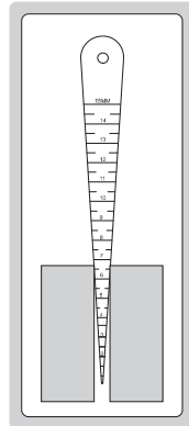
楔形塞尺测量缝隙宽度
